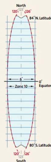
UTM slice, Zone 10. Longitude red, UTM grid in blue
